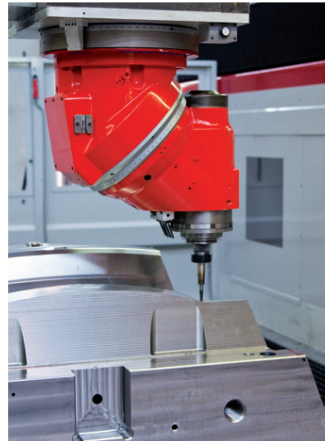
Hochgeschwindigkeitsbearbeitung von Spritzgussformen für Stoßfänger in der Automobilindustrie
