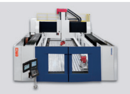
Dynamill HP5 mit mechanischem Fräskopf und 5-Achs-Fräskopf mit Elektrospindel X= 12.050 mm Y= 4.000 mm Z= 1.500 mm
